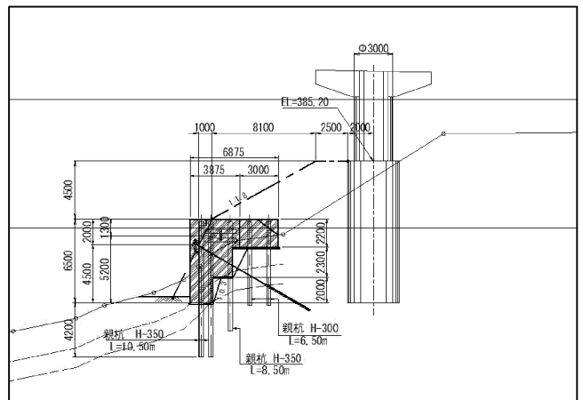
図-4 山留式擁壁断面図
