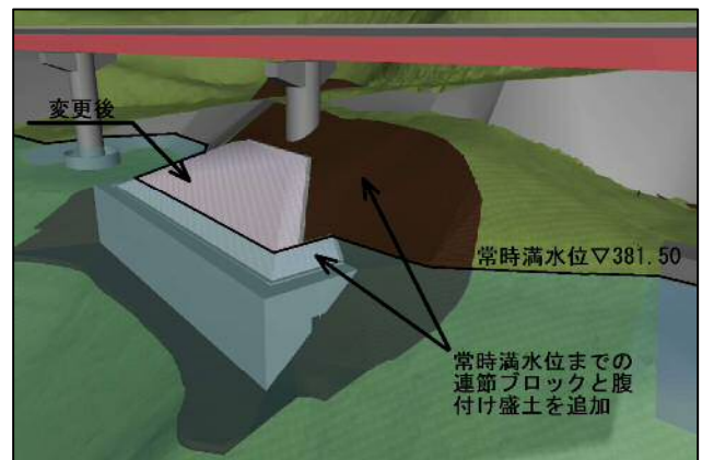
図-8 変更後 3Dモデル
