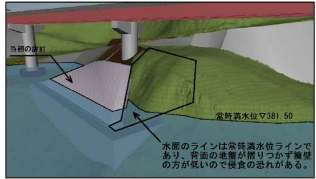
図-7 3Dモデルによる検証
