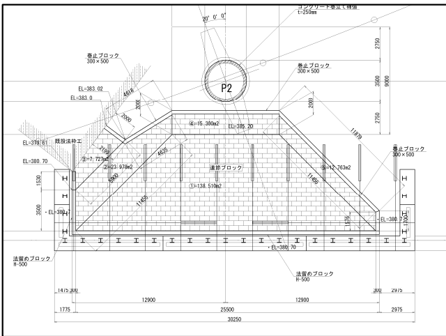
図-6 連節ブロック平面図
